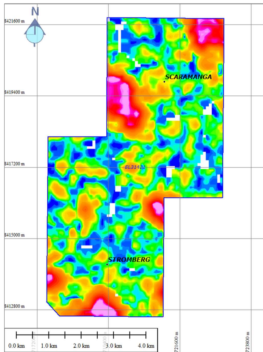
MAG: TMI-RTP-AS image
