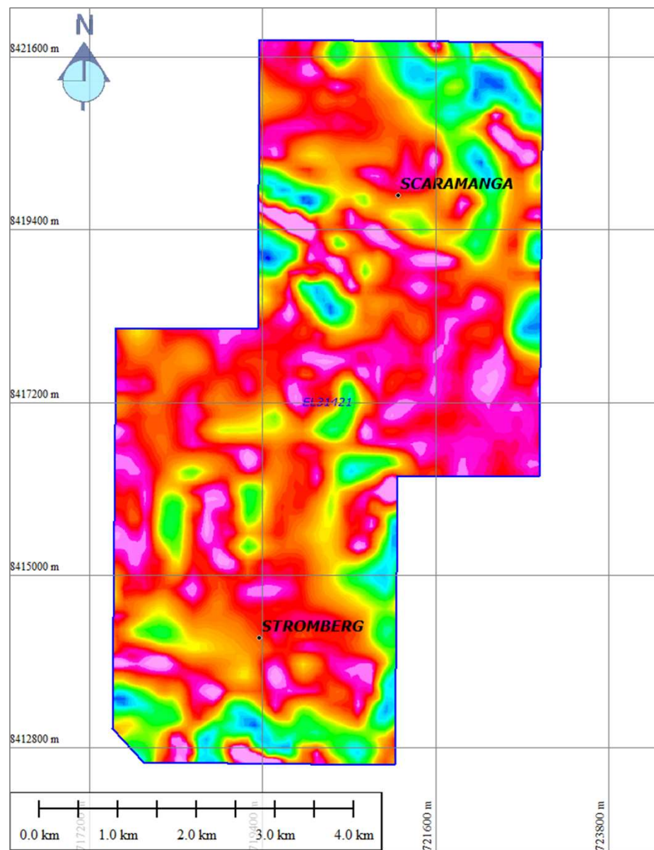
MAG: TMI-RTP-1VD image
